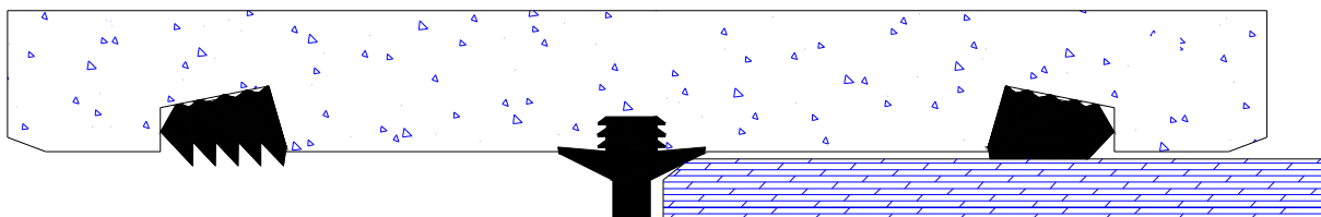
Sección del manguito con detalle de la junta elastomérica y el stopper
